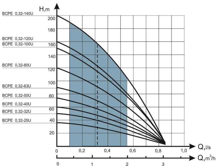
Obr. 2 Tlakové charakteristiky čerpadla
