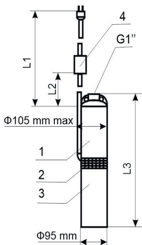
Obr.1 Rozmery a pripojovacie rozmery
