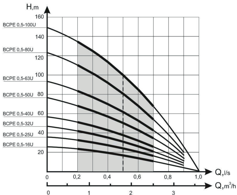
Obr. 2 Tlakové charakteristiky čerpadla
