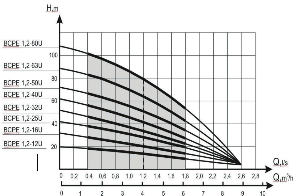
Obr. 2 Tlakové charakteristiky čerpadla
